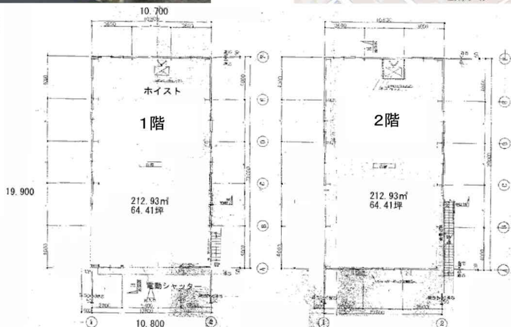
【平面図】
